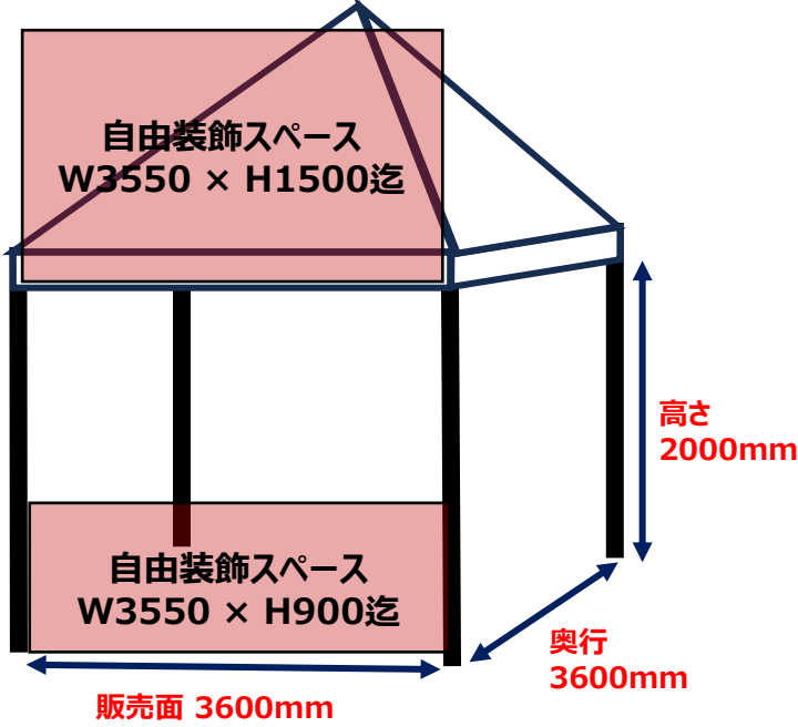
【立面図】
