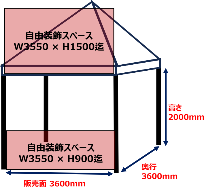
【立面図】
